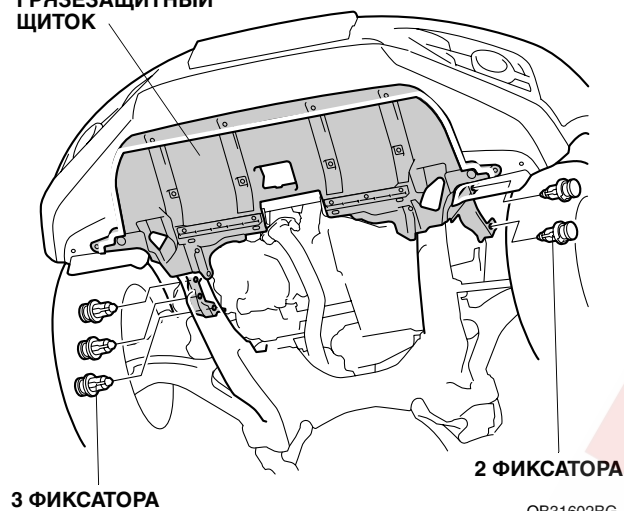
ГРЯЗЕЗАЩИТНЫЙ ЩИТОК
